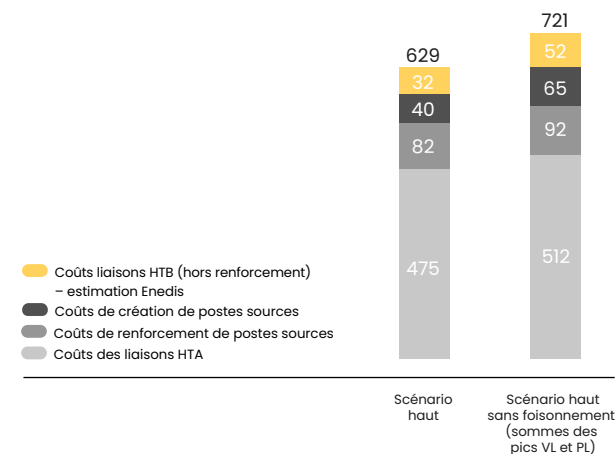
Figure 21 : Investissements requis sur le réseau électrique avec et sans foisonnement des besoins de recharge des VL et des PL, aire par aire
